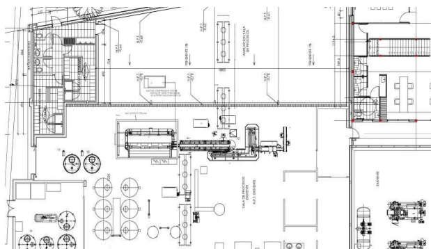
PIANTA/DISEGNO TECNICO DELL'OFFICINA
